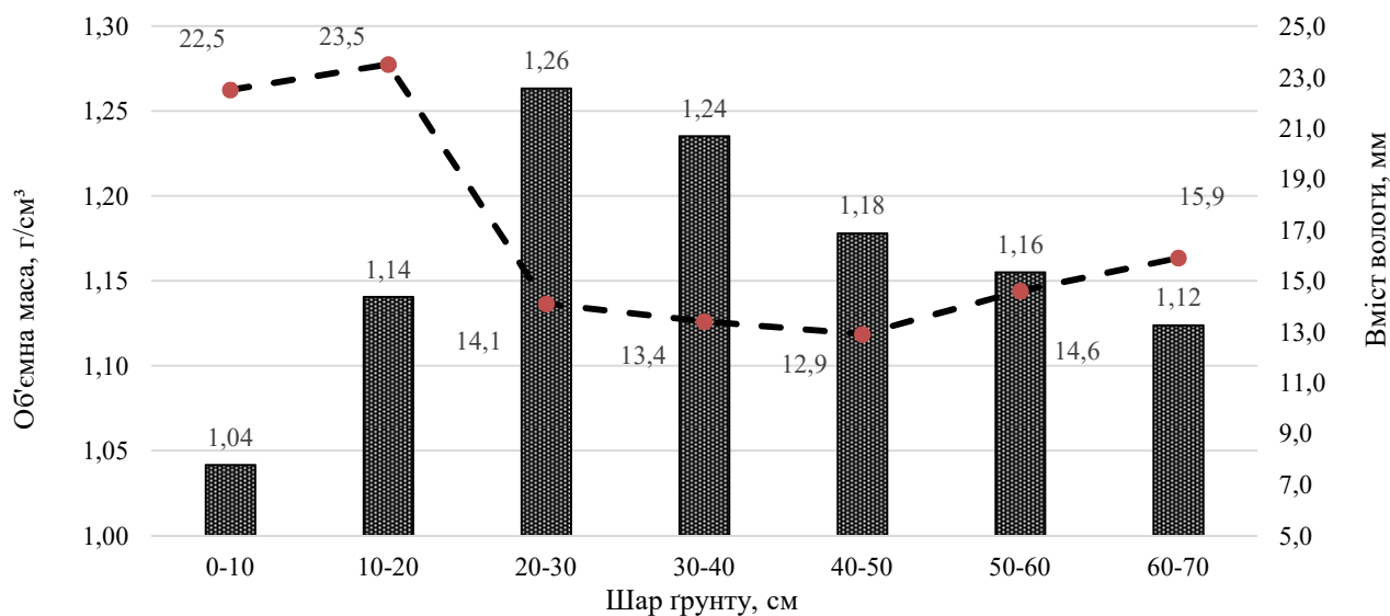
Рис. 1. Вміст води в ґрунті залежно від його щільності за традиційної технології обробітку ґрунту в осінній період 2015 р.
